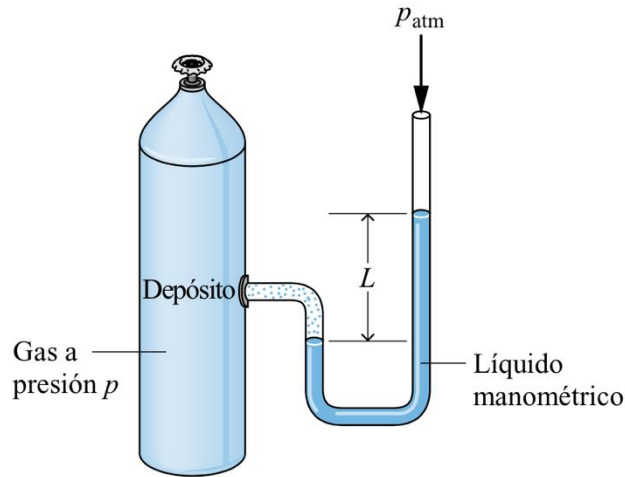
Figura 1.3.2. Medida de la presión con un manómetro (Moran y Shapiro 2004).
