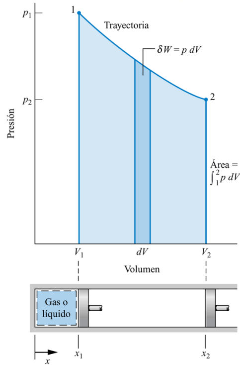
Figura 1.3.2. Trabajo de un proceso cuasiestático de expansión en un diagrama p-V (Moran y Shapiro 2004).
