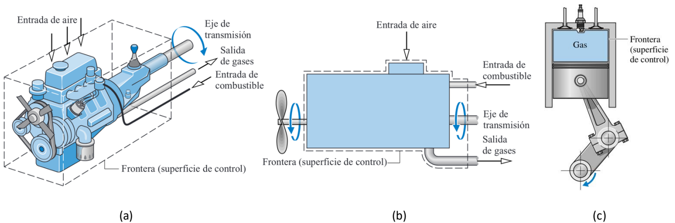
Figura 1.3.1. Diferentes tipos de sistemas: (a) el motor de un coche (sistema abierto), (b) su sección transversal y (c) el gas contenido en un pistón que lo compone (sistema cerrado) (adaptación de Moran y Shapiro 2004).
