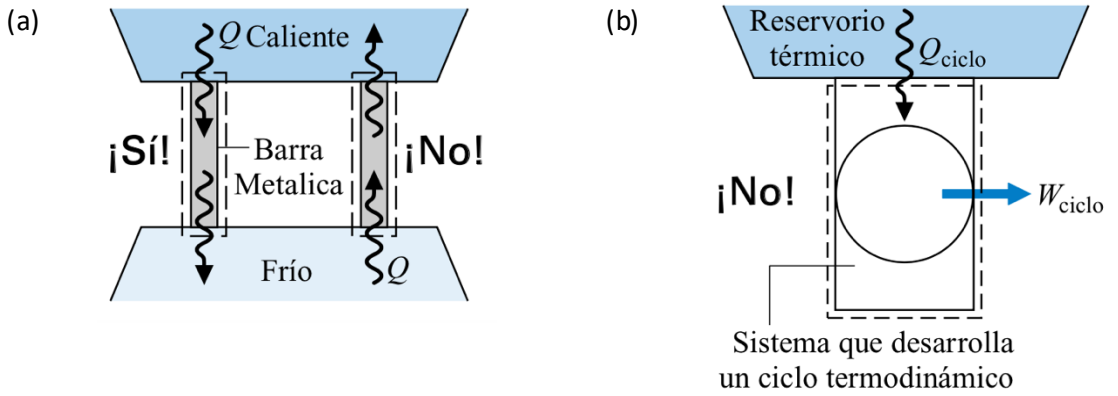
Figura 1.2.2. Formulaciones del segundo principio de la Termodinámica según (a) Clausius y (b) Kelvin-Planck (Moran y Shapiro 2004).
