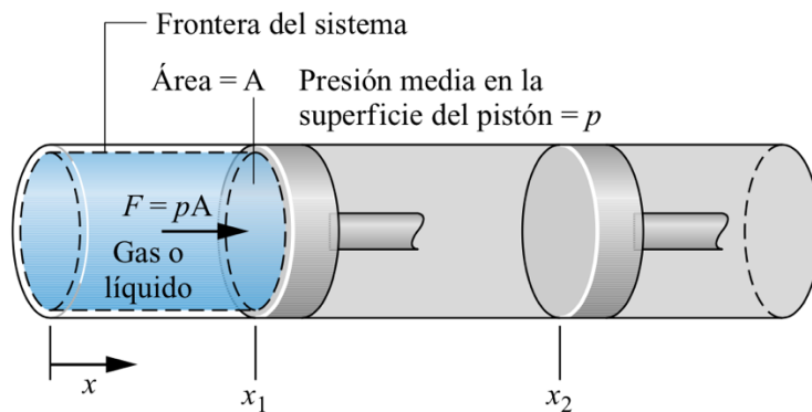
Figura 1.3.4. Expansión o compresión de un gas o un líquido (Moran y Shapiro 2004).
