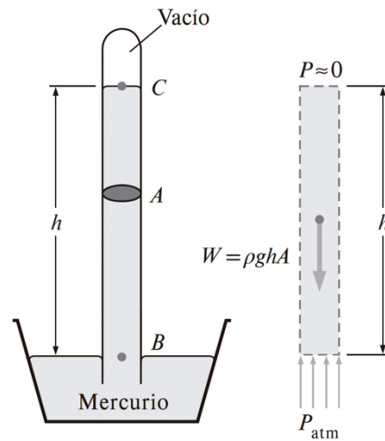
Figura 1.3.3. Barómetro básico basado en el experimento de Torricelli (Çengel 2019).
