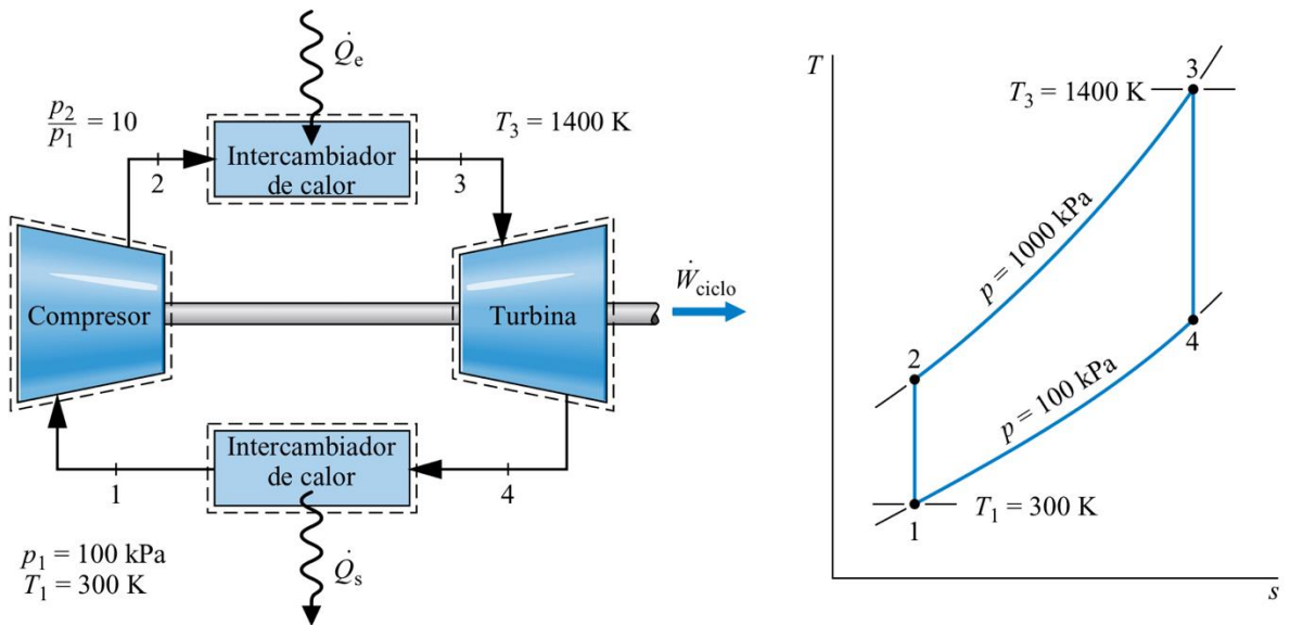
Figura 1.3.3. Proceso de un ciclo Brayton de aire estándar y su diagrama T-s (Moran y Shapiro 2004).
